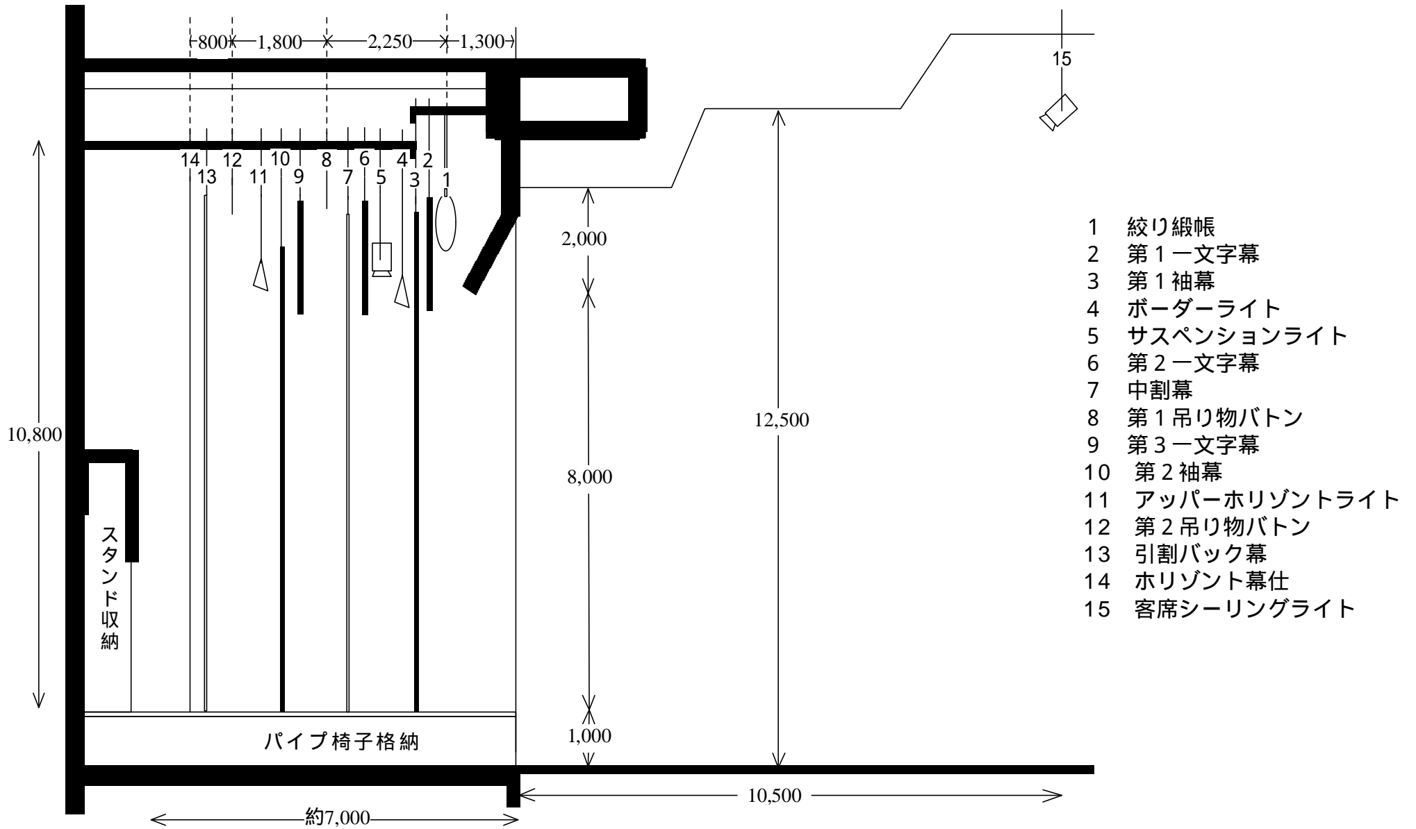
「上山市体育文化センター アリーナ」舞台吊物装置配置図
